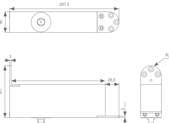
parte inferior de la puerta - posición angular
