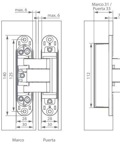
invisible neo L-7 resistente al fuego
