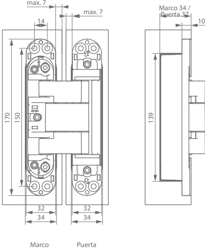
invisible neo L-7 resistente al fuego
