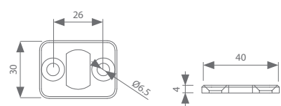
pieza de anclaje al suelo
