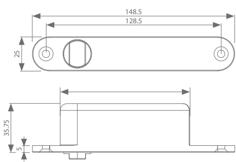
pieza superior de anclaje a la hoja de la puerta
