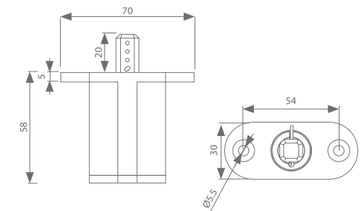
pieza de anclaje inferior en la hoja de la puerta
