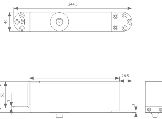
parte inferior de la puerta - posición central o descentrada
