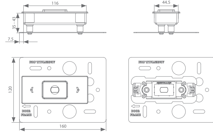
parte inferior del suelo - empotrado (=bi)
